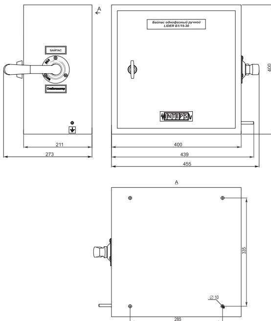
Габаритные и установочные размеры байпаса однофазного ручного LIDER Б 1/15-30
