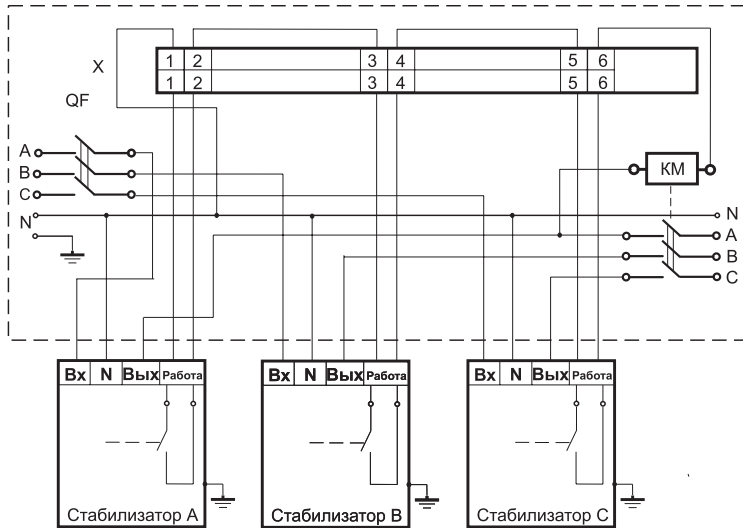
QF - трехфазный автоматический выключатель KM - трехфазный контактор
